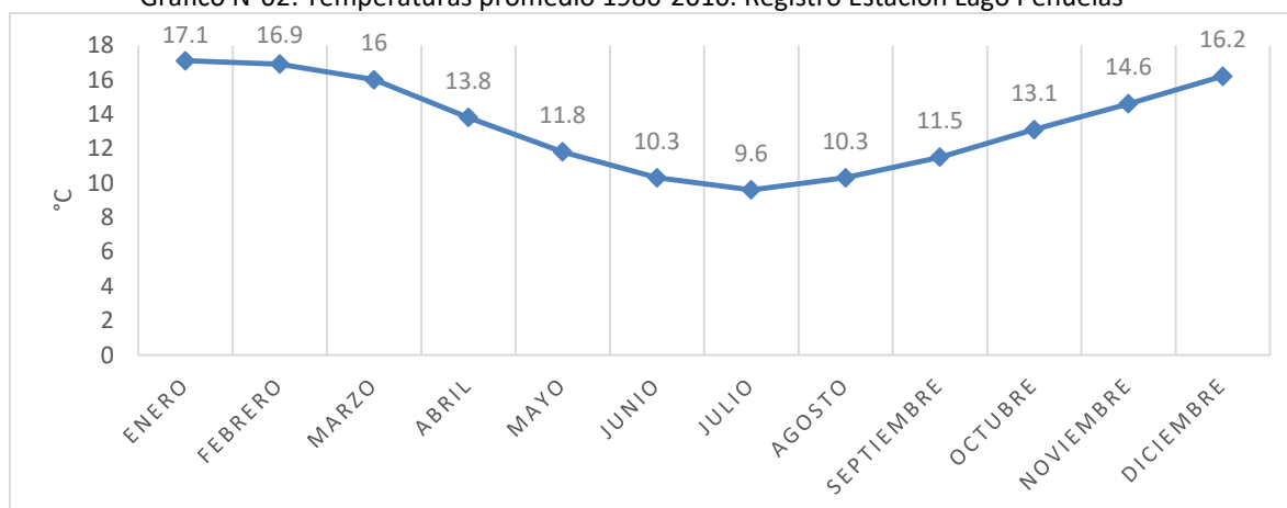
Grafico N°02: Temperaturas promedio 1980-2010. Registro Estación Lago Peñuelas
